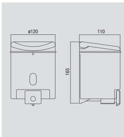
Ref: 1575 00 Dosificador de jabón Soap dispenser PVP: 35,00 € Caja - Box / carton 1/12
