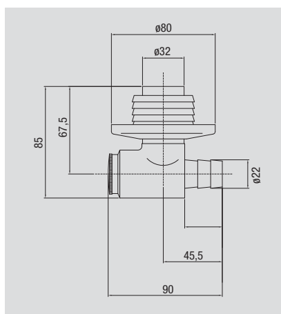
Ref: 1629 07 Sifón botella para lavadora Chromed trap for washing-machine PVP: 11,50 € Caja - Box / carton 1/45
