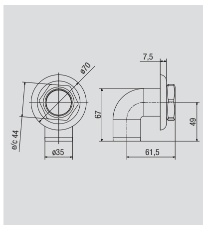
Ref: 1630 06 / 07 Curva técnica Technical bend PVP: 8,00 € Caja - Box / carton 4/80
