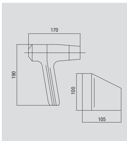
Ref: 1786 220V / 1786 110V Secador de cabello con soporte Hair dryer with holder PVP: 33,50 € Caja - Box / carton 1/18
